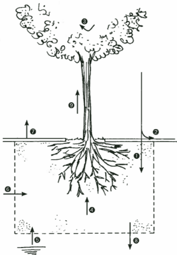
Schema van de watercyclus bij stadsbomen: 1. infiltratie van neerslag 2. afstromen van het oppervlak 3. verdamping vanuit bladeren. 4. opname vanuit grondwater 5. capillaire opstijging vanuit grondwater 6. zijdelingse aanvoer grondwater 7. verdamping vanaf bovengrond 8. uitzijging naar grondwater 9. vochtopname en verdamping van het water in de boom (bron: stadsbomenvademecum deel 2A)
